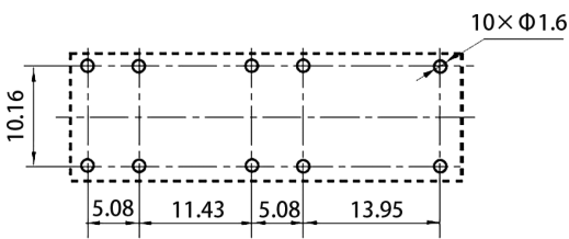
安装孔尺寸 (底视图)
